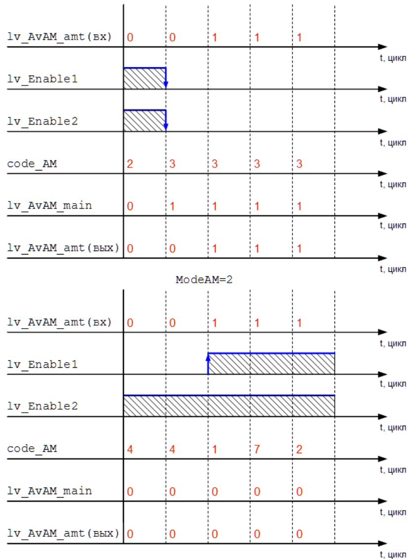
Рисунок 3 – Временная диаграмма ввода резерва.
