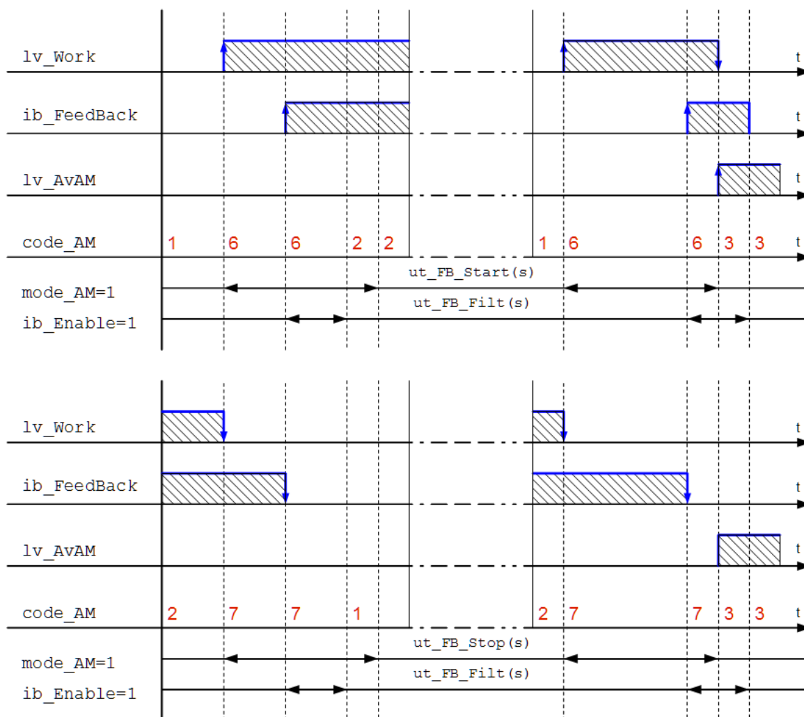
Рисунок 2 – Временная диаграмма
