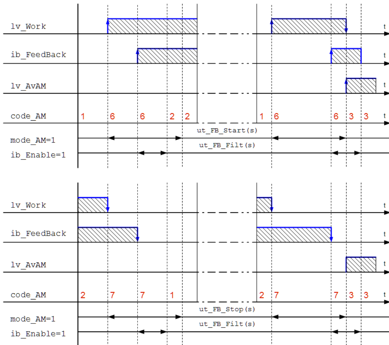
Рисунок 8 – Временная диаграмма
