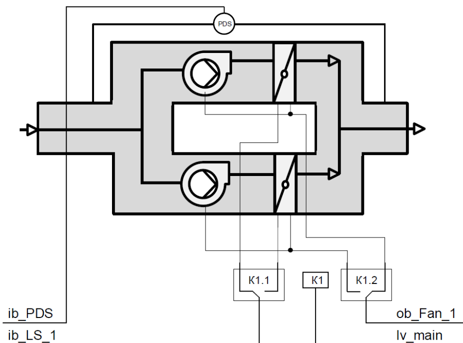
Рисунок 3 – Схема подключения для режима 1.
