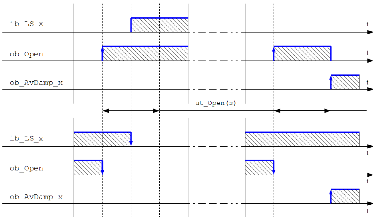
Рисунок 9 – Временная диаграмма.
