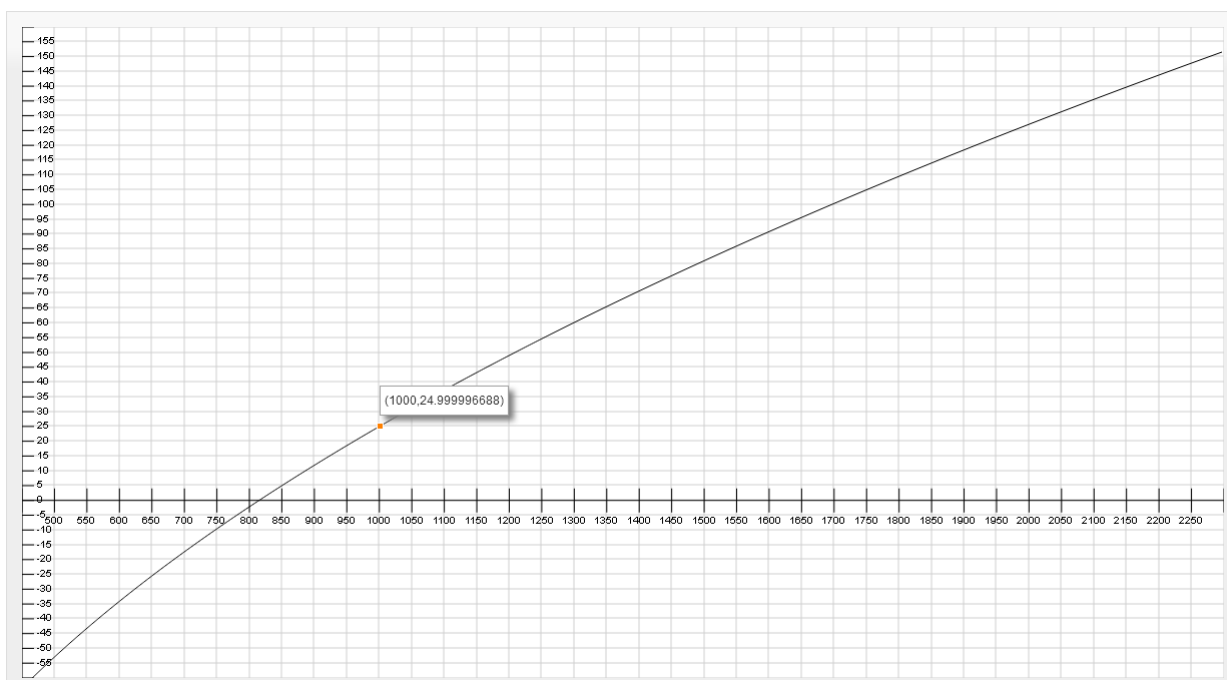
Рисунок 2 – График для вычисления температуры из сопротивления датчика Для удобства использования макроса и проверки его работы, приведена таблица преобразования сопротивления в температуру.
