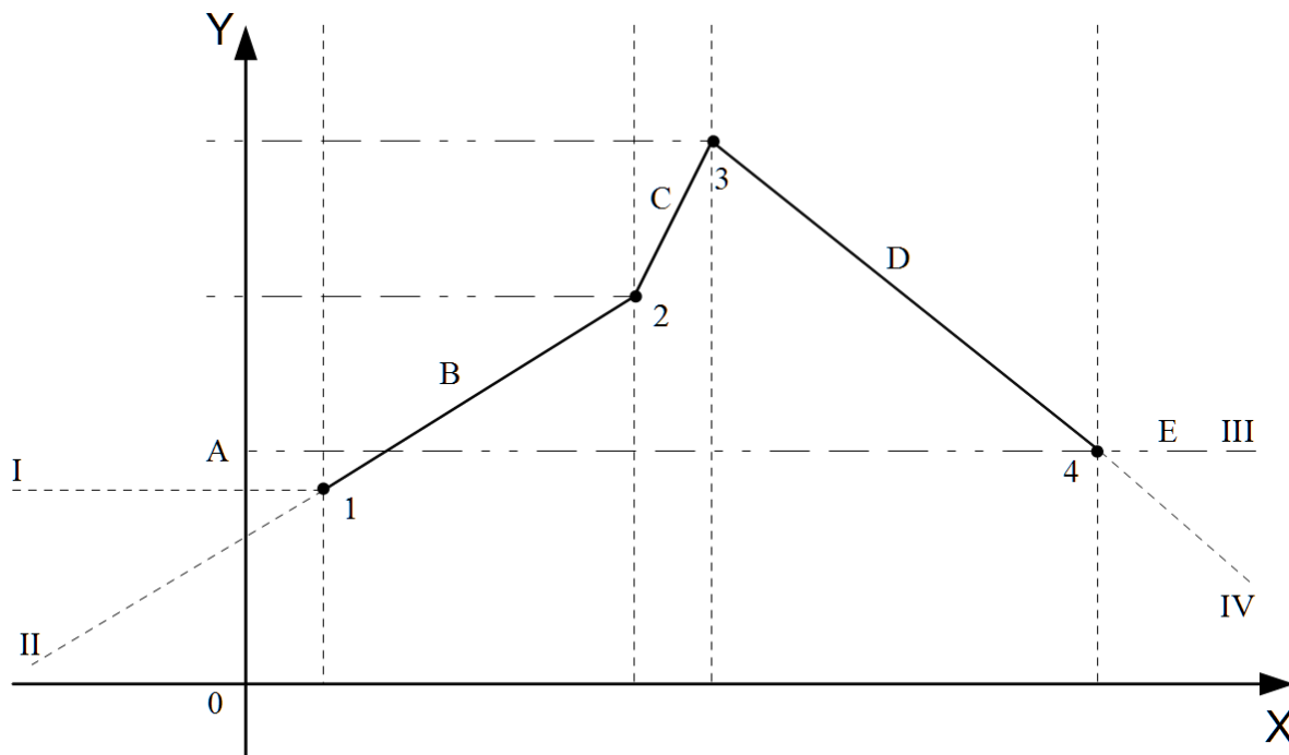
Рисунок 2 – Пример вычисления
